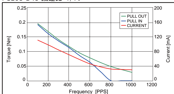
PG25S-D48 減速比 1/76
