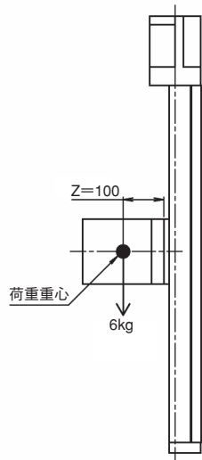
荷重分布図
