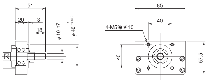
モータ取付部形状：RN
