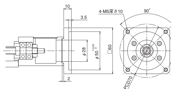
モータ取付部形状：B1（質量：37g）
