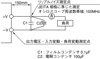
特性測定回路
