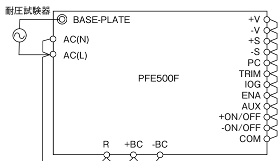
図21-1 入力ベースプレート間耐電圧試験方法
