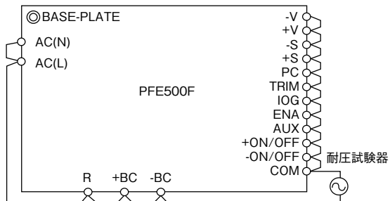
図21-2 入力出力間耐電圧試験方法
