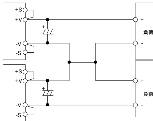
図11-2 土出力使用の直列運転
