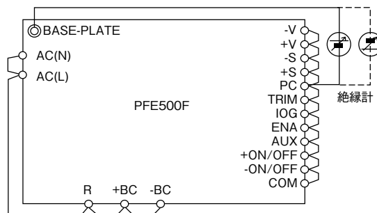
図22-1 絶縁抵抗試験方法
