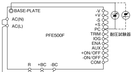
図21-3 出力ベースプレート間耐電圧試験方法
