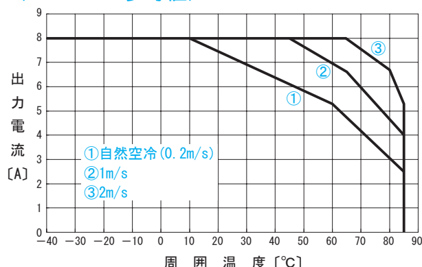
●CHS200483R3 出力ディレーティング特性 ( V_{in}=48V 参考値)
