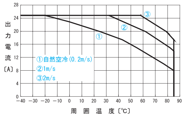
●CHS3004812H 出力ディレーティング特性 ( V_{in}=48V 参考値)
