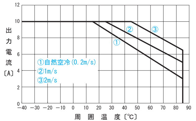
●CHS1202412 出力ディレーティング特性 ( V_{in}=24V 参考値)
