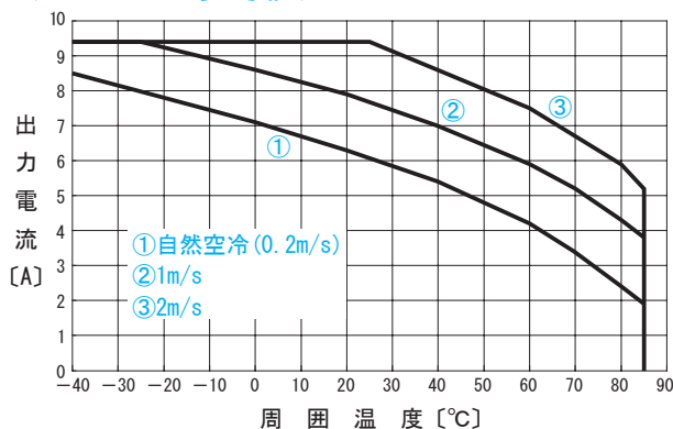
●CHS3004832 出力ディレーティング特性 ( V_{in}=48V 参考値)
