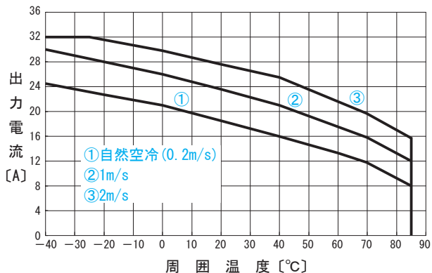
●CHS3804812 出力ディレーティング特性 ( V_{in}=48V 参考値)
