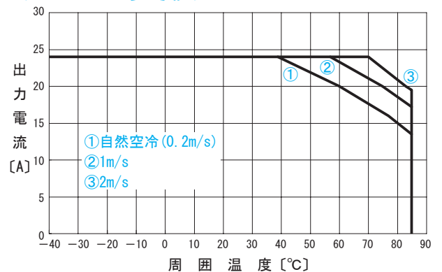
●CHS1204805 出力ディレーティング特性 ( V_{in}=48V 参考値)
