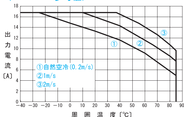
●CHS3002412 出力ディレーティング特性 ( V_{in}=24V 参考値)
