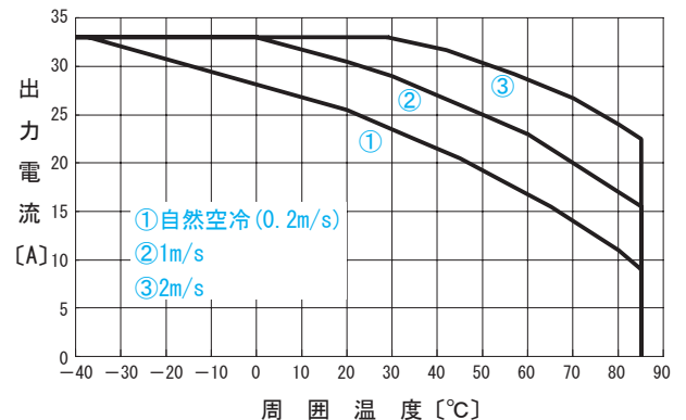
●CHS4004812 出力ディレーティング特性 ( V_{in}=48V 参考値)
