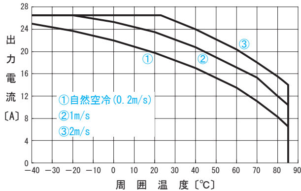
●CHS4002424 出力ディレーティング特性 ( V_{in}=24V 参考値)
