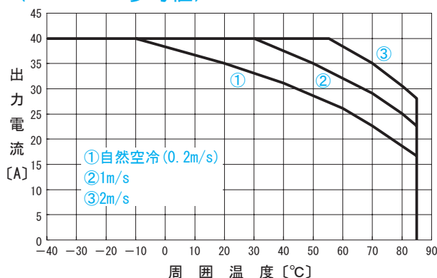
●CHS3002405 出力ディレーティング特性 ( V_{in}=24V 参考値)
