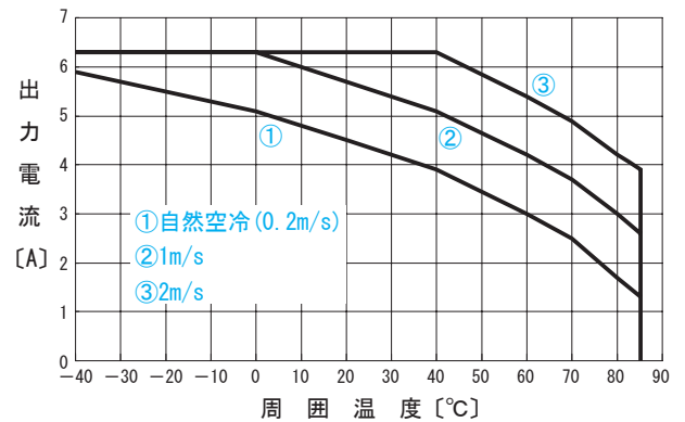
●CHS4002448 出力ディレーティング特性 ( V_{in}=24V 参考値)
