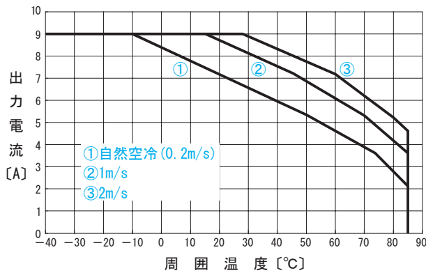
●CHS3002428 出力ディレーティング特性 ( V_{in}=24V 参考値)
