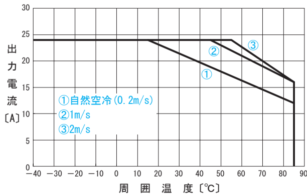
●CHS1202405 出力ディレーティング特性 ( V_{in}=24V 参考値)
