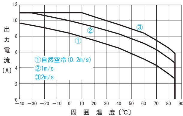
●CHS4002432 出力ディレーティング特性 ( V_{in}=24V 参考値)
