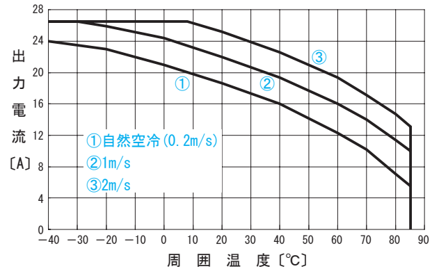
●CHS4002428 出力ディレーティング特性 ( V_{in}=24V 参考値)
