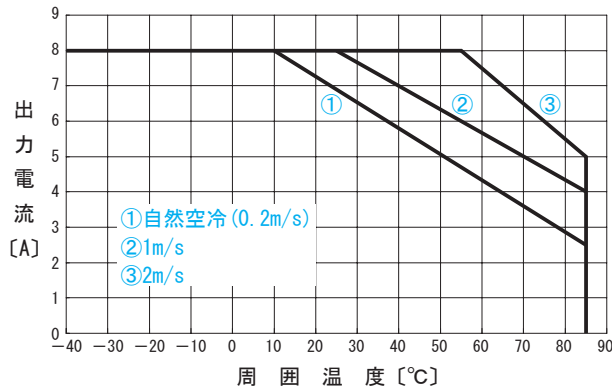
●CHS1202415 出力ディレーティング特性 ( V_{in}=24V 参考値)
