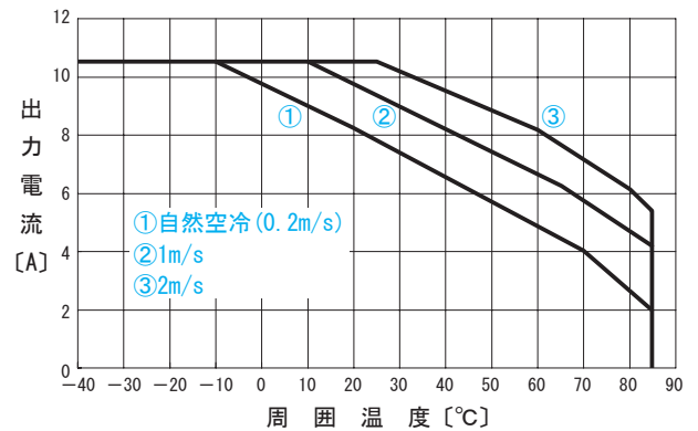
●CHS3002424 出力ディレーティング特性 ( V_{in}=24V 参考値)
