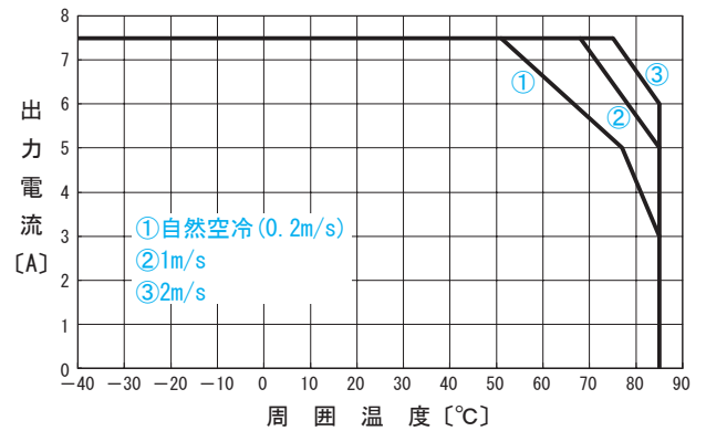
●CHS804812 出力ディレーティング特性 ( V_{in}=48V 参考値)
