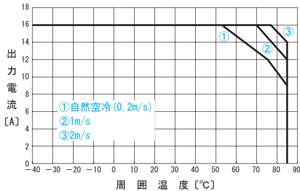
●CHS804805 出力ディレーティング特性 ( V_{in}=48V 参考値)
