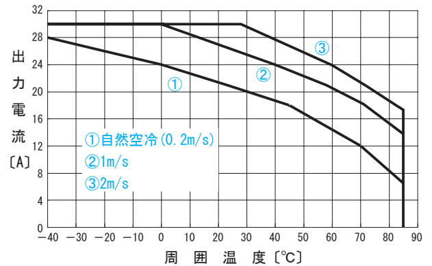
●CHS3004810 出力ディレーティング特性 ( V_{in}=48V 参考値)
