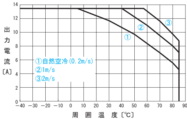
●CHS3002415 出力ディレーティング特性 ( V_{in}=24V 参考値)
