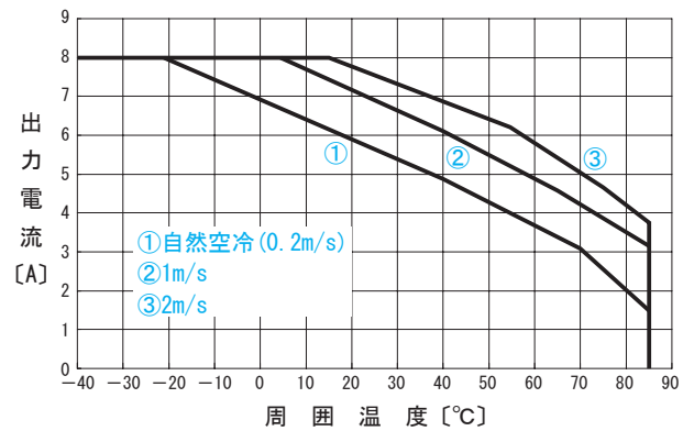
●CHS3002432 出力ディレーティング特性 ( V_{in}=24V 参考値)
