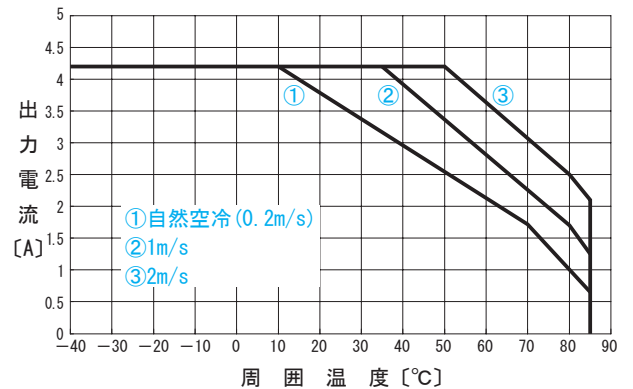
●CHS1202424 出力ディレーティング特性 ( V_{in}=24V 参考値)
