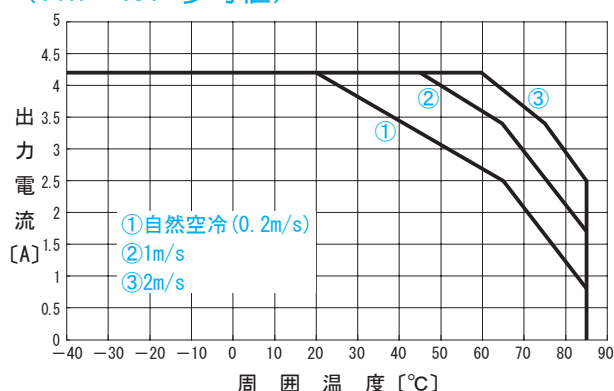
●CHS1204824 出力ディレーティング特性 ( V_{in}=48V 参考値)
