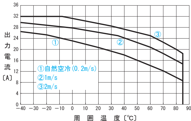
●CHS3804812H 出力ディレーティング特性 ( V_{in}=48V 参考値)
