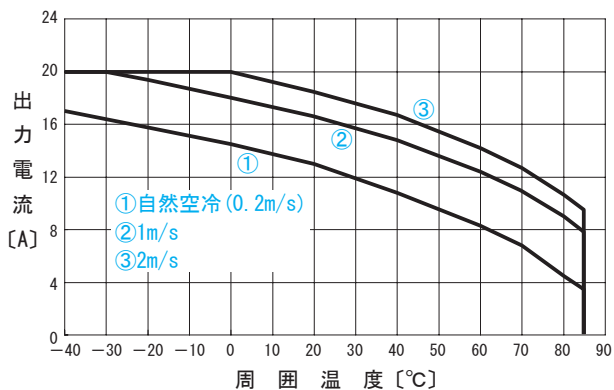
●CHS3004828 出力ディレーティング特性 ( V_{in}=48V 参考値)
