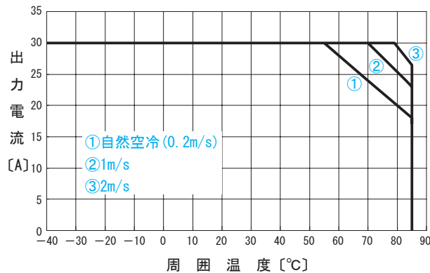
●CHS120483R3 出力ディレーティング特性 ( V_{in}=48V 参考値)
