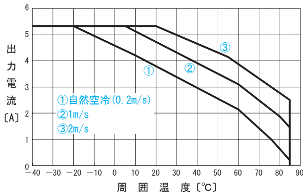
●CHS3002448 出力ディレーティング特性 ( V_{in}=24V 参考値)
