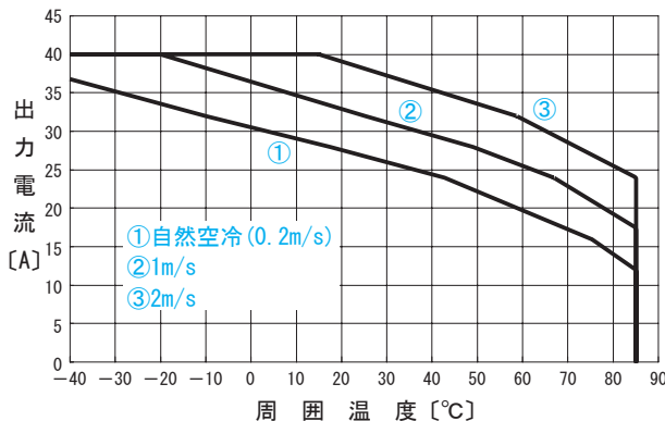
●CHS4004810 出力ディレーティング特性 ( V_{in}=48V 参考値)
