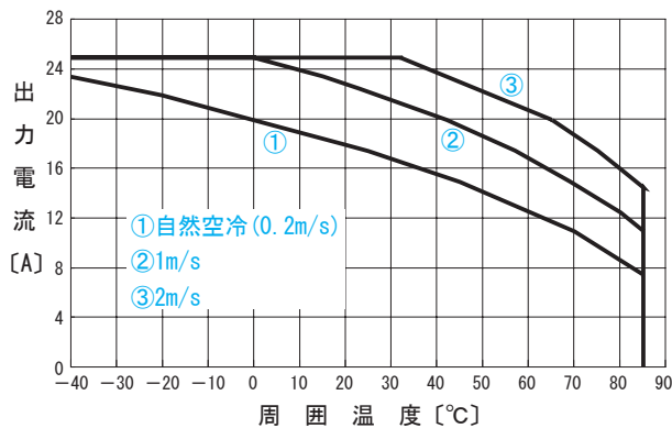
●CHS3004812 出力ディレーティング特性 ( V_{in}=48V 参考値)
