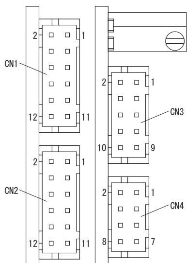
コネクタピン番号
