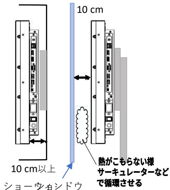
側面
